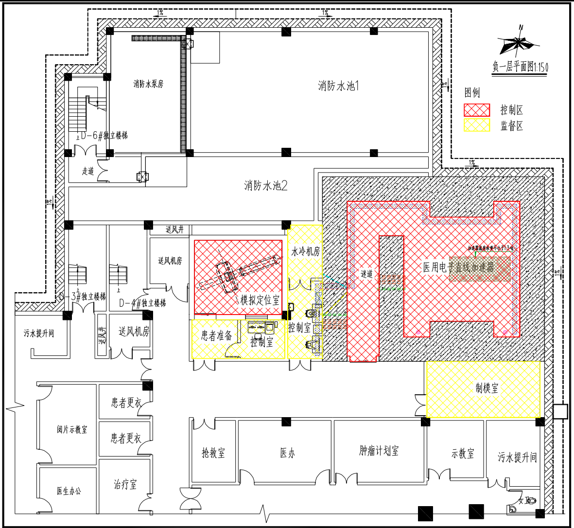
图 10-1 肿瘤科分区示意图
