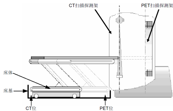
图 9-7 PET/CT 结构示意图
