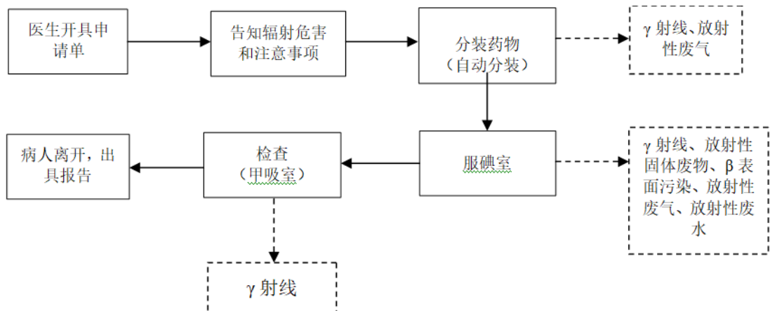
图 9-12 ^{131}\text{I} 甲状腺吸碘功能测定项目工作流程及产污环节分析示意图
