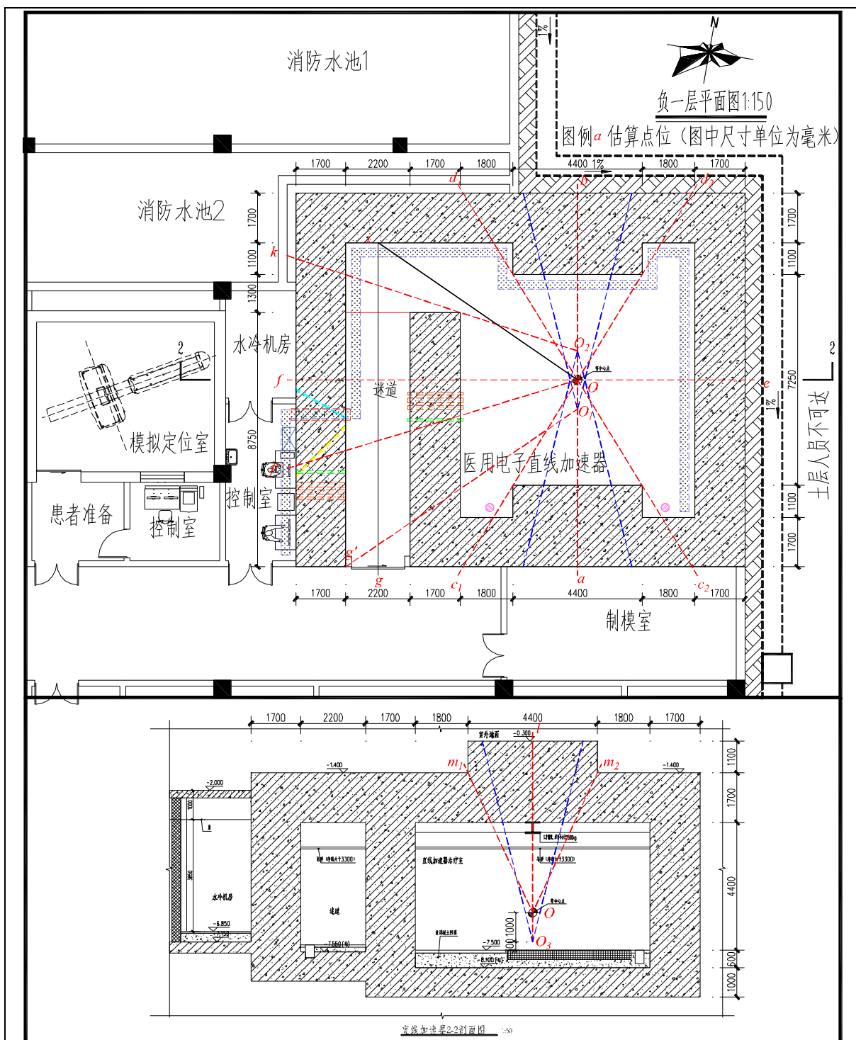
图 11-1 医用电子直线加速器机房关注点位置示意图
