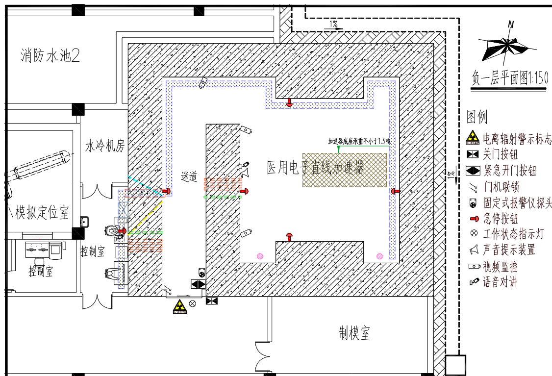
图 10-5 本项目医用电子直线加速器机房辐射安全设施布置示意图
