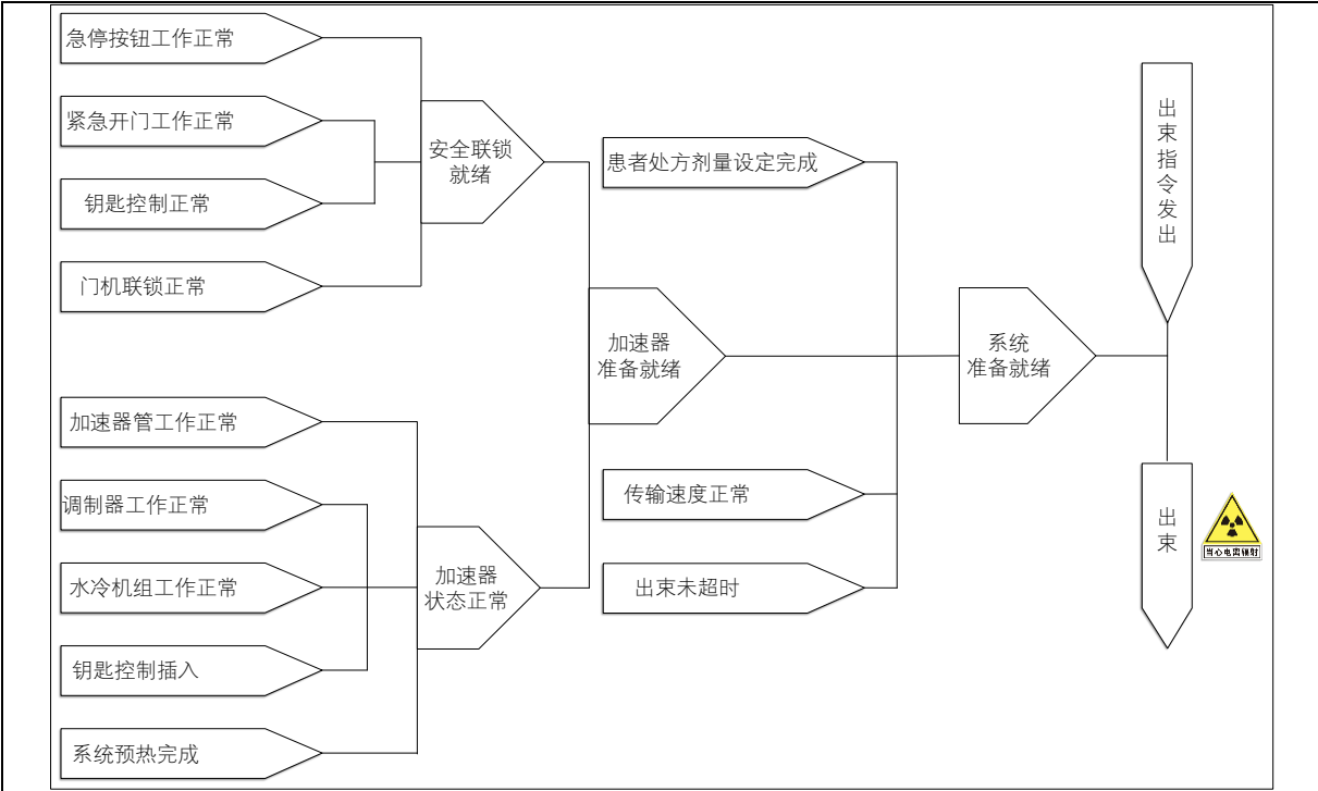
图 10-6 医用电子直线加速器安全联锁逻辑示意图
