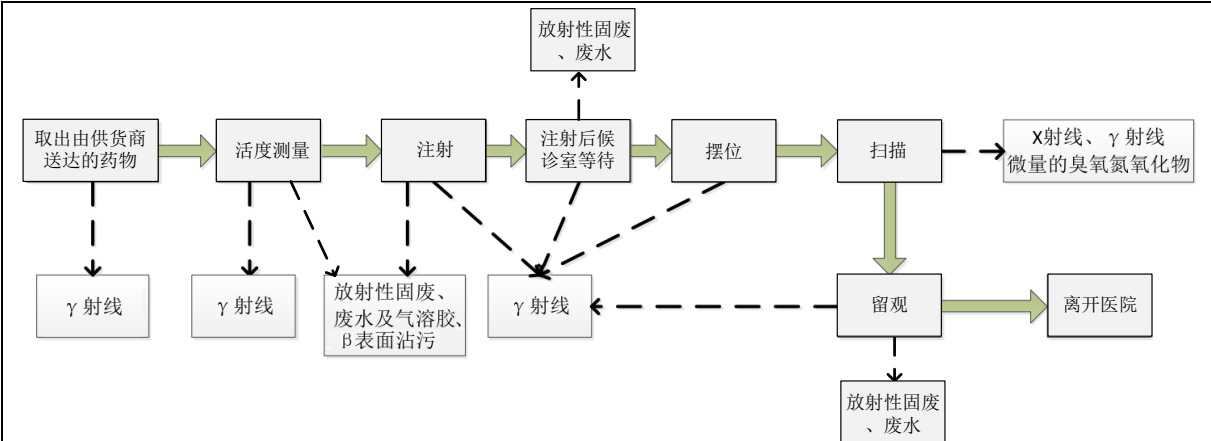
图 9-11 SPECT/CT 诊断项目工作流程及产污环节分析示意图
