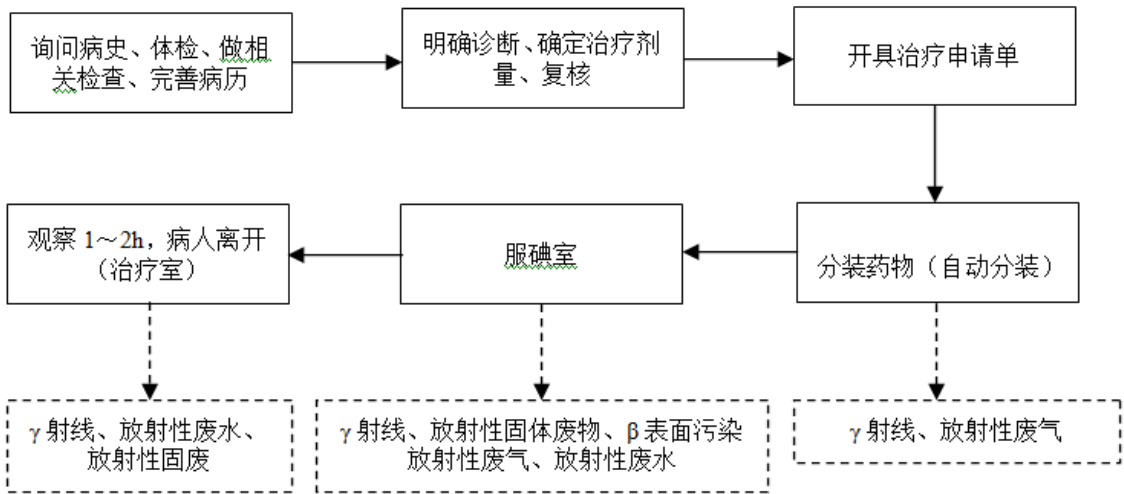
图 9-13 ^{131}\text{I} 甲亢治疗项目工作流程及产污环节分析示意图
